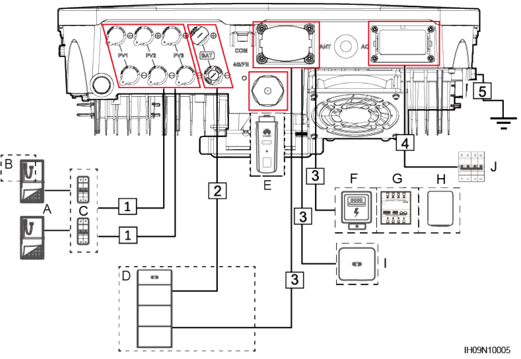
Figure 5-1 Connexions des câbles du SUN2000 (les composants dans l'encadré en pointillé sont facultatifs)
