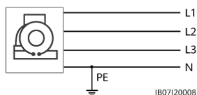
Figure 5-6 Mise à la terre des fils neutres du générateur
