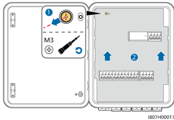
Figure 5-5 Ouverture du couvercle du compartiment de maintenance
