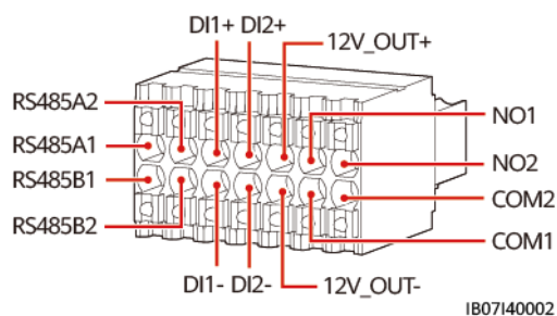
Figure 5-22 Définitions des broches
