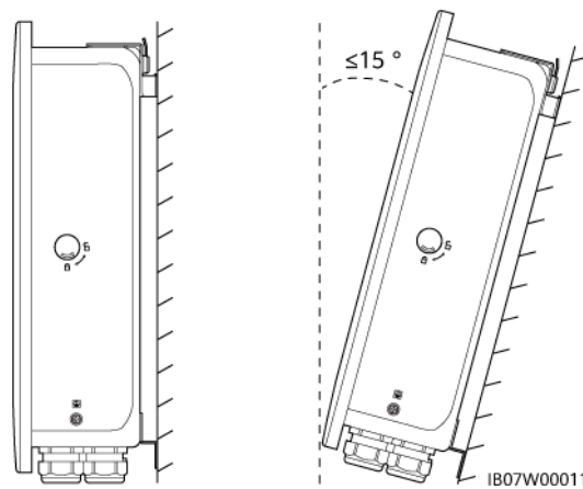
Figure 4-3 Angle d'installation
