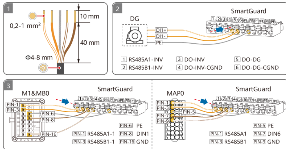
Figure 5-18 Sertissage des bornes d'extrémité de cordon pour le câble de signal (la case en pointillée indique un composant facultatif)
