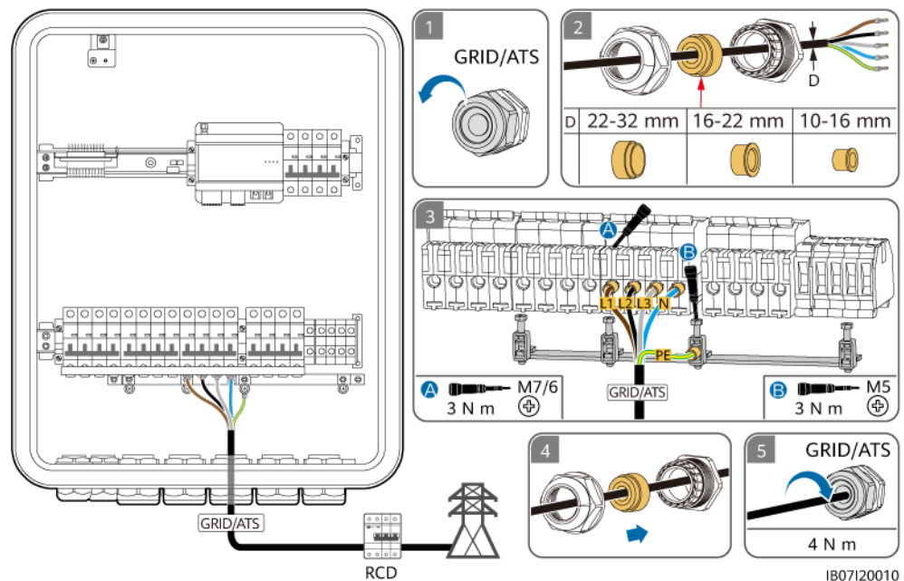
Figure 5-8 Connexion du câble d'alimentation de sortie CA du réseau
