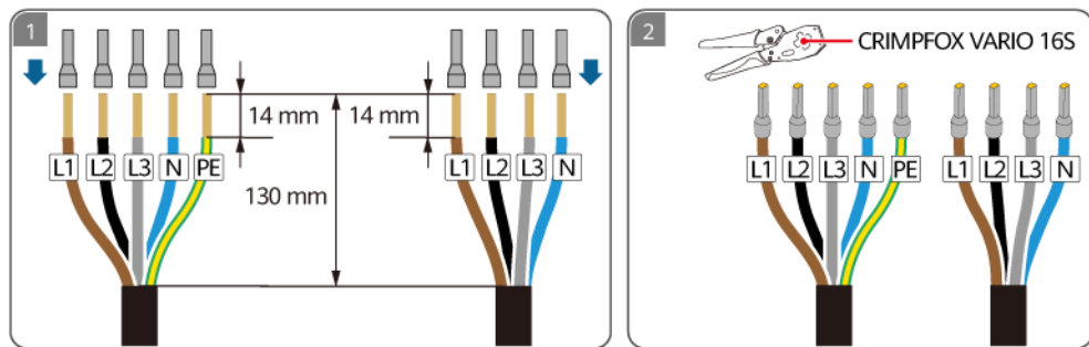
Figure 5-10 Sertissage des bornes d'extrémité du cordon CA
