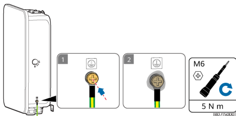
Figure 5-3 Connexion du câble PE
