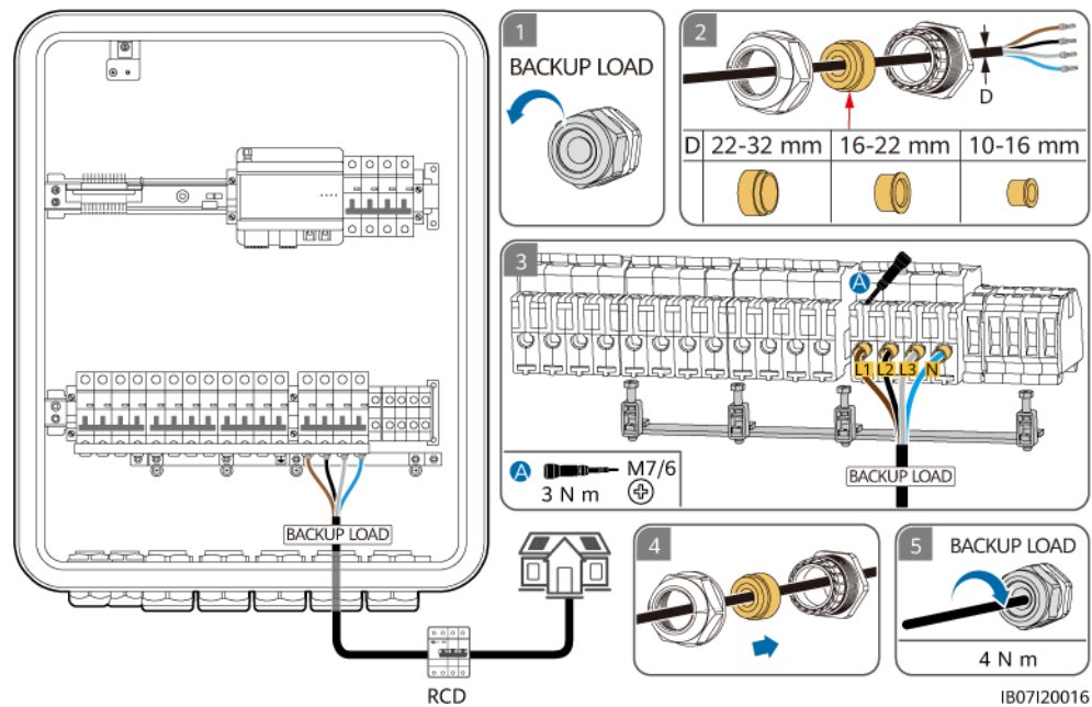
Figure 5-15 Connexion du câble d'alimentation de la charge de secours du SmartGuard-63A-AUTO
