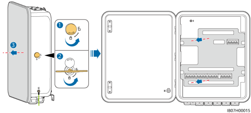
Figure 5-4 Ouverture de la porte du compartiment de maintenance
