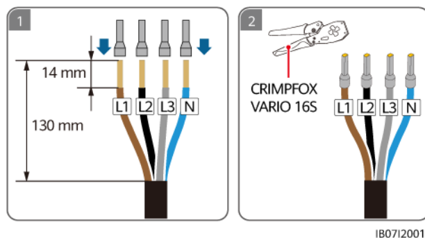
Figure 5-13 Sertissage des bornes d'extrémité du cordon CA pour le SmartGuard-63A-AUTO
