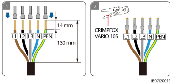
Figure 5-12 Sertissage des bornes d'extrémité du cordon CA pour la SmartGuard-63A-T0
