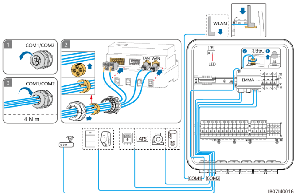
Figure 5-26 Connexion des câbles de signal EMMA (les cases en pointillés indiquent les composants facultatifs)
