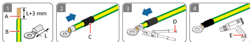
Figure 5-2 Sertissage d'une borne OT
