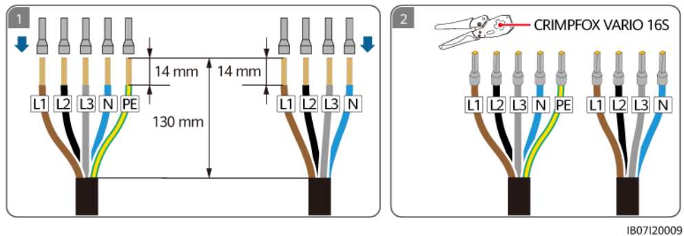
Figure 5-16 Sertissage des bornes d'extrémité du cordon CA
