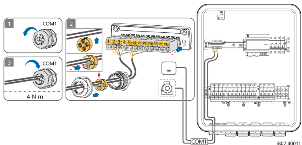
Figure 5-20 Connexion des câbles de signaux du SmartGuard (la case en pointillée indique un composant facultatif)
