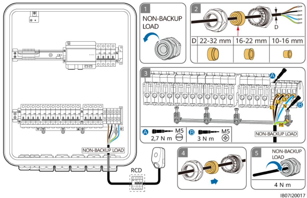
Figure 5-17 Connexion du câble d'alimentation de sortie sans charge de secours (la case en pointillés indique un composant facultatif)
