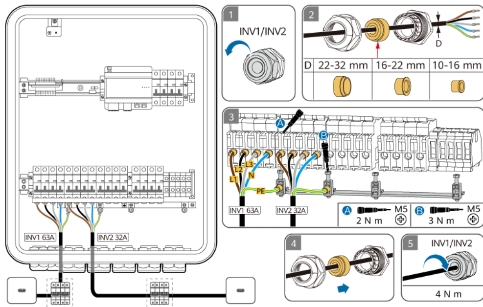
Figure 5-11 Branchement des câbles d'alimentation d'entrée CA de l'onduleur (cases en pointillés indiquant les composants facultatifs)
