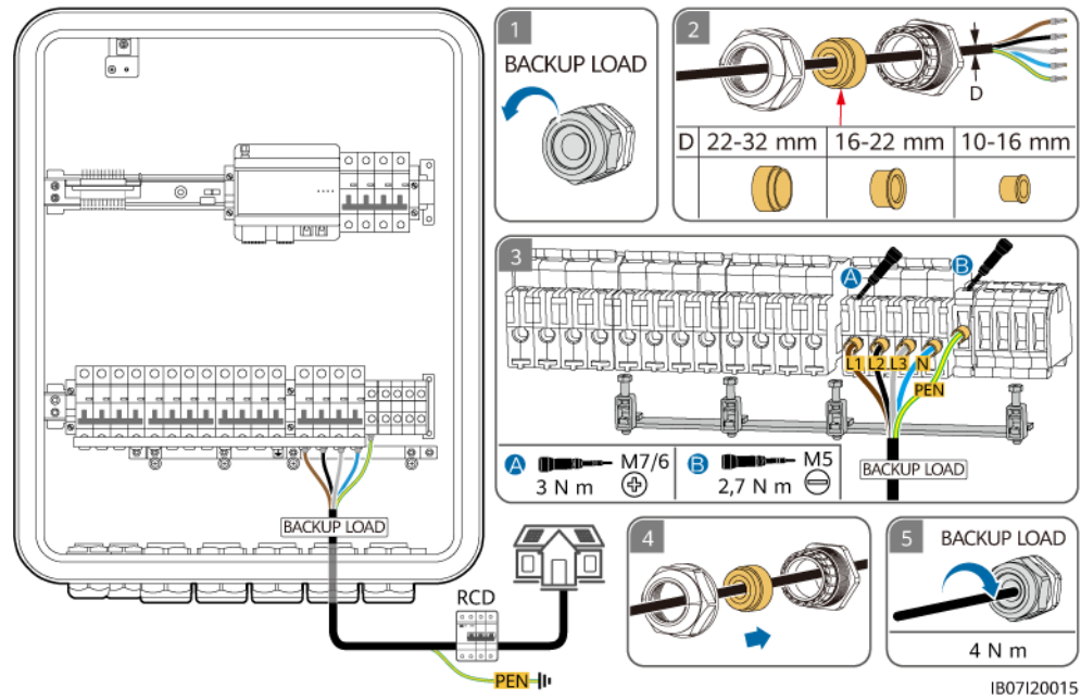
Figure 5-14 Connexion du câble d'alimentation de la charge de secours du SmartGuard-63A-T0
