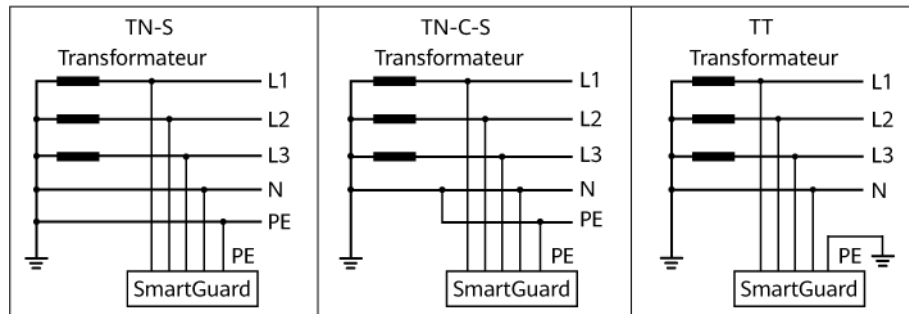
Figure 2-7 Systèmes de mise à la terre
