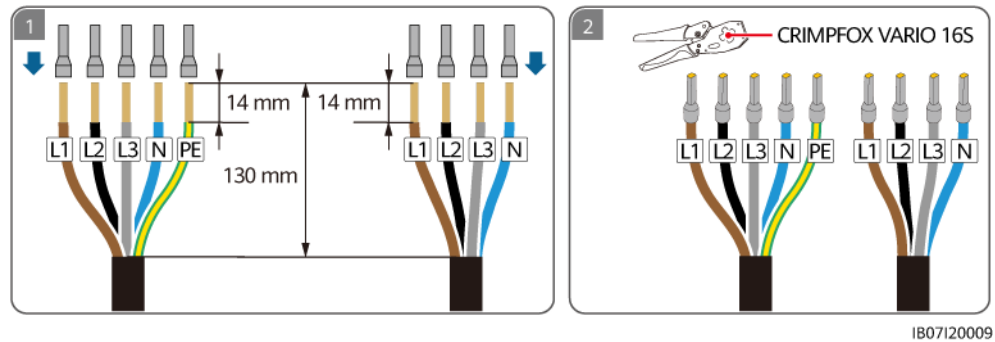
Figure 5-7 Sertissage des bornes d'extrémité du cordon CA
