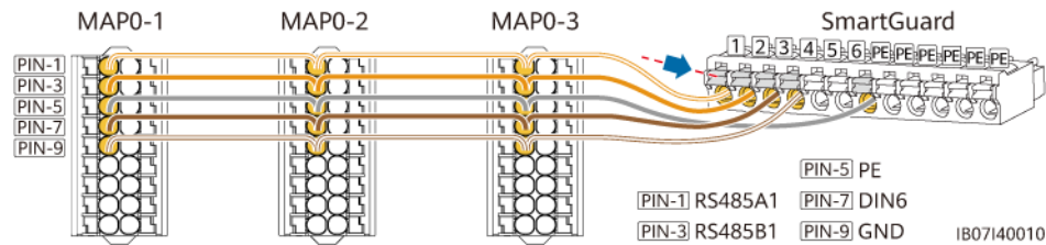
Figure 5-19 Connexion parallèle de câbles de signaux (en utilisant trois onduleurs connectés en parallèle à titre d'exemple)
