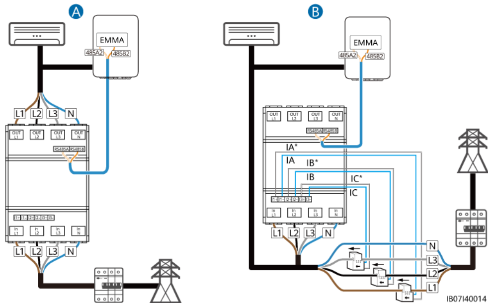
Figure 5-24 Connexion du câble de communication du compteur électrique
