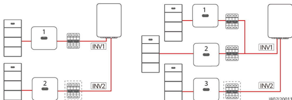
Figure 5-9 Onduleurs MAP0 connectés en parallèle (les cases pointillées indiquent les composants facultatifs)
