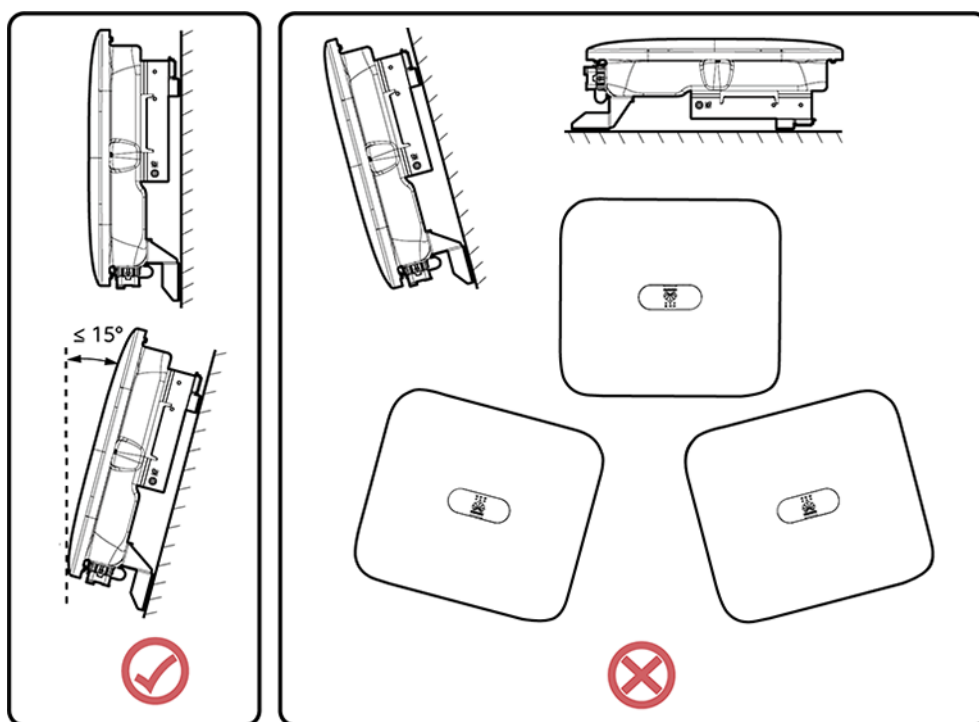
Figure 4-1 L'installation s'incline
