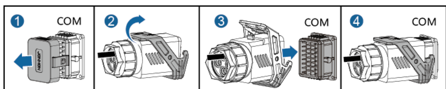
Figure 5-33 Fixation du connecteur du câble de signal
