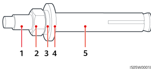
Figure 4-8 Composition d'un boulon à expansion
