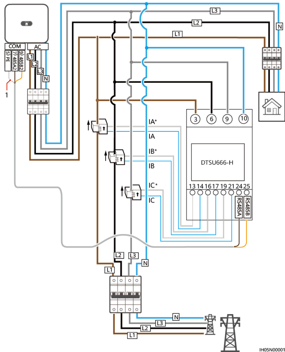
Figure 5-24 Connexion de câble (triphasé, quatre câbles)
