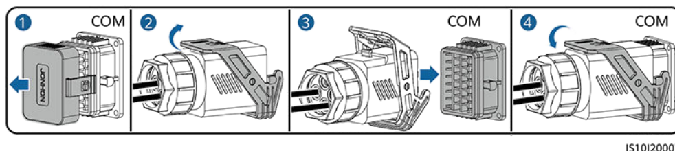
Figure 5-28 Fixation du connecteur du câble de signal
