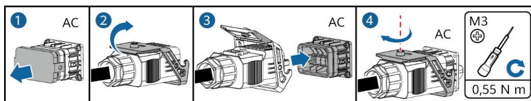
Figure 5-9 Fixation d'un connecteur CA
