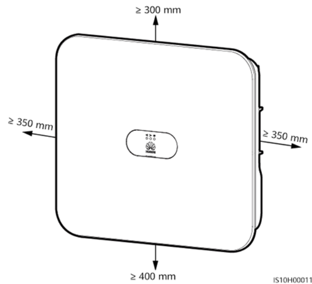
Figure 4-2 Espace d'installation
