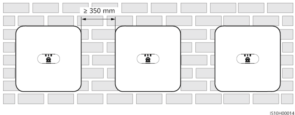
Figure 4-3 Installation horizontale (recommandée)
