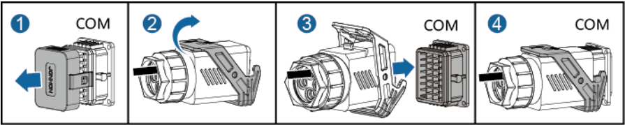
Figure 5-26 Fixation du connecteur du câble de signal
