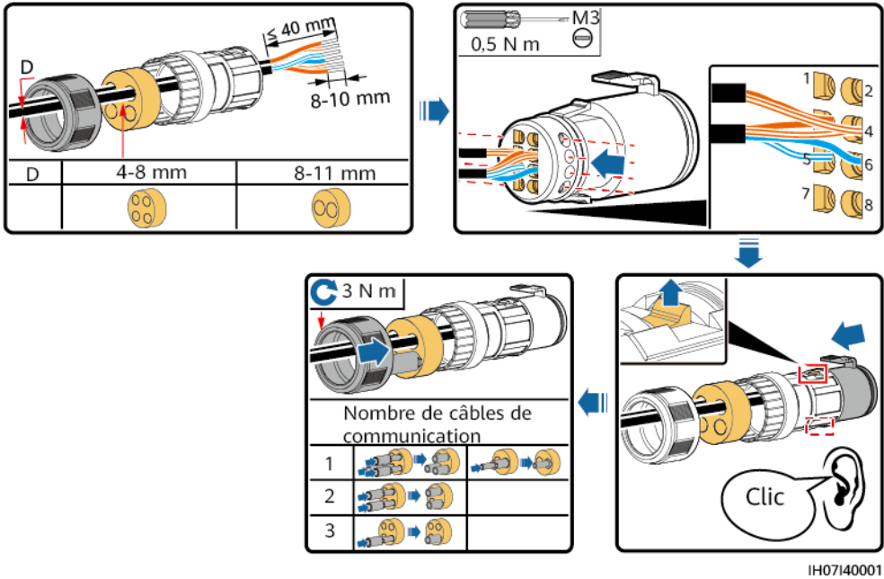
Figure 5-25 Assemblage d'un connecteur de signal (SUN2000 simple)
